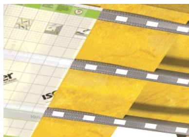
Obr. 2 ISOVER VARIO® XtraPatch aplikovaná na sádkartonovú podkonštrukciu.
