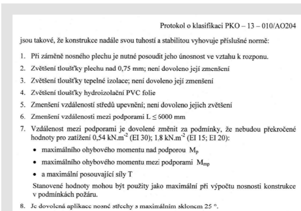
Obr. 8: Statická časť požiarnej klasifikácie, s ktorou je spojené závadné Uistenie o požiarnej odolnosti.
